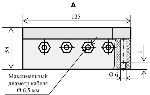
Рисунок 1 - Блок P485
